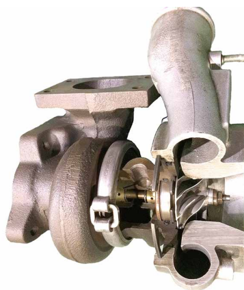
▲ターボチャージャー
