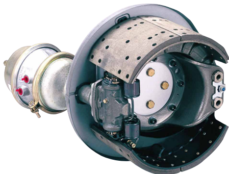
▲ドラムブレーキ
